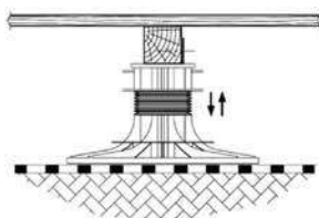
8 platelages (lames + lambourdes) sur plots géotextiles et sol brut stabilisés
